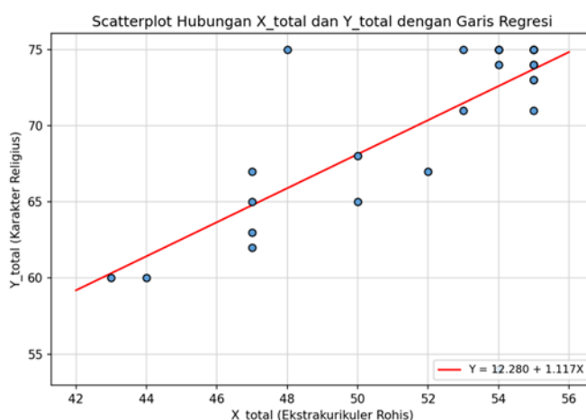
Gambar 4. Scatterplot Hubungan X_total dan Y_total dengan Garis Regresi
